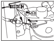
Moottori- kopan lukitus vaijeri (oikea)
