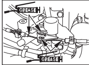
Moottori- kopan lukitus- vaijeri (vasen)
