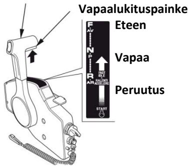
Kaukosäätövipu
